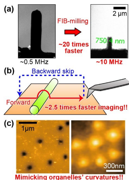
図 1：(a) FIBによって作成された超小型カンチレバー。(b) Only-trace-imaging モード。(c) 凹面／凸面基板。
