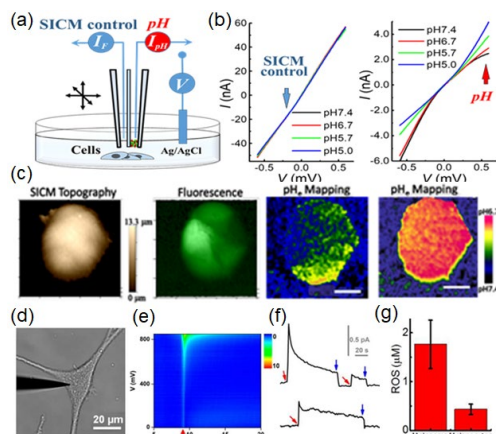
図 4 : (a) SICMと細胞外pH(pHe)の同時イメージングの概略図。(b) pHナノプローブは、pHセンシングとサンプルとの距離制御が可能なる2つのバレルを有する。(c) CD44 GFP MCF7細胞のSICMおよび蛍光イメージングとpHeマッピング。(d) 細胞内に挿入したナノプローブの光学画像。(e) ROS計測のためのナノプローブによるメラノーマ細胞内のサイクリックボルタンメトリー。(f) ナノプローブによるメラノーマ内部(赤矢印)と外部(青矢印)のROS由来の電流計測。(g) メラノーマおよびメラノサイト内のROS濃度の違い。
